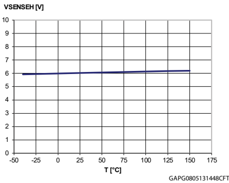
Figure 34: Vsenseh vs. Tcase
